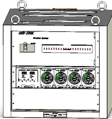
OSR-200K(정류기)
